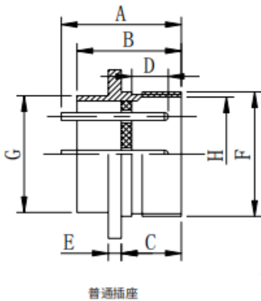
Размерная схема серии Авиационный разъем CX 2 стандартный
