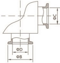
KF法兰
