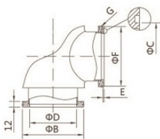
GB-LP法兰
