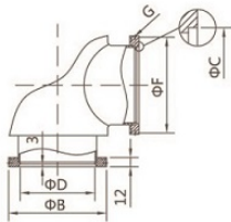
LF法兰
