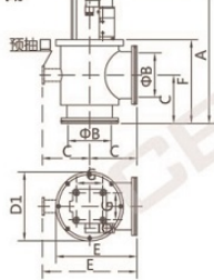
DN 63~250 气动
