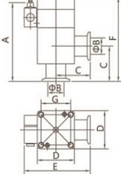
DN16~50 铝阀体 气动
