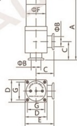
DN16~50 铝阀体 电磁
